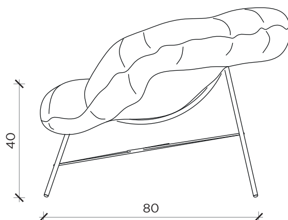
LATO | SIDE
