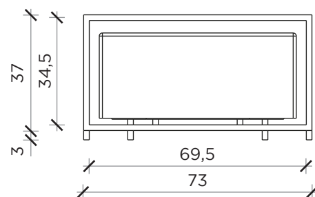
LATO | SIDE
